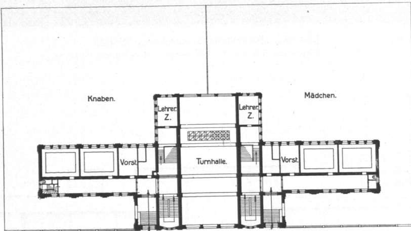
Abb. 231. Volksschule Bullenhuser Damm, Erdgeschoss.
