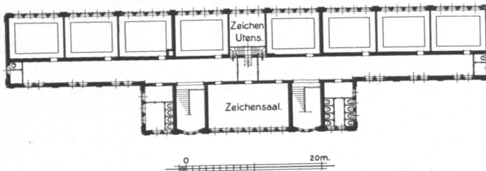
Abb. 232. Volksschule Bullenhuser Damm, Obergeschoss.
