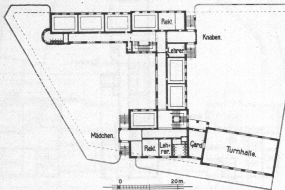
Abb. 220. Volksschule Morahntstraße, Erdgeschoss.
