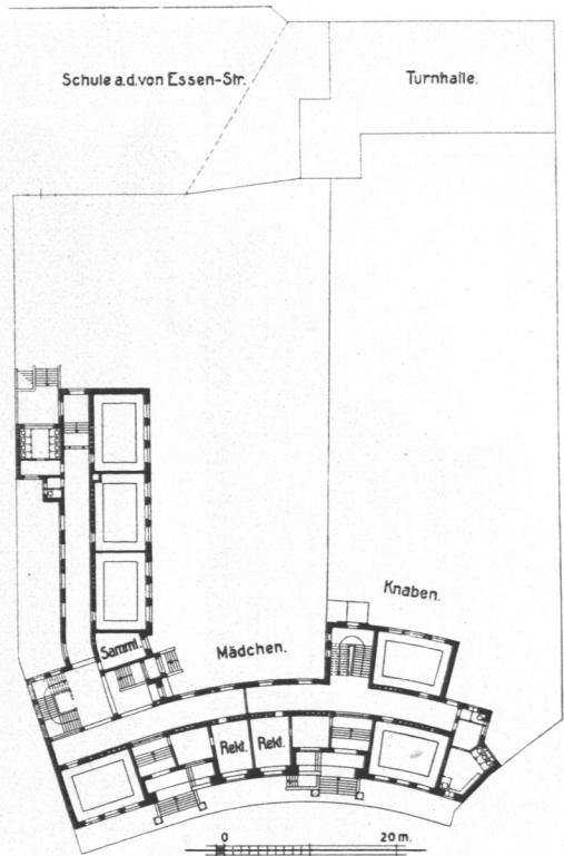
Abb. 208. Volksschule von Essenstraße, Erdgeschoß.
