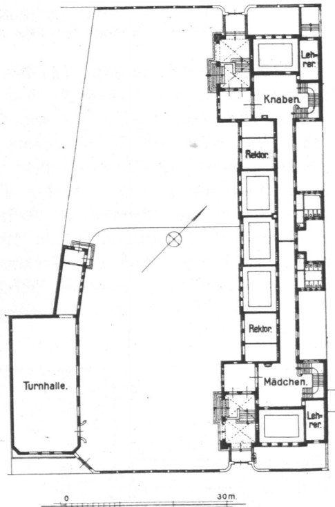
Abb. 210. Volksschule Telemannstraße, Erdgeschoß.
