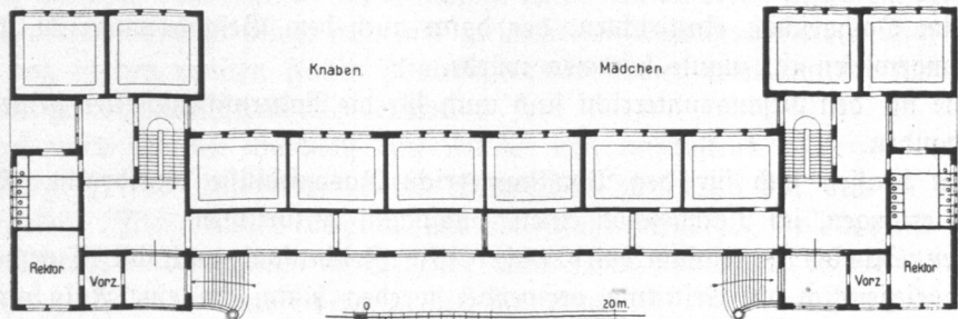
Abb. 206. Volksschule Käthnerkamp, Erdgesch. Hof.
