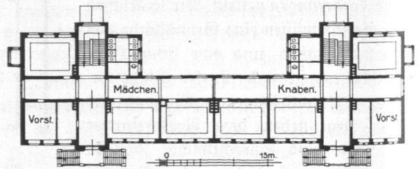
Abb. 204. Volksschule Ausschlägerweg, Erdgesch. Hof.
