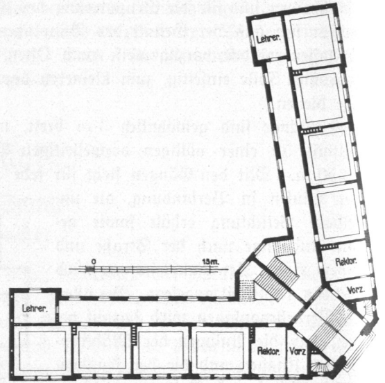
Abb. 202. Volksschule Kantstraße und Schellingstraße, Erdgesch. Hof.
