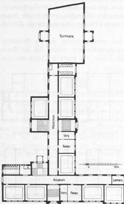
Abb. 203. Volksschule Reginenstraße, Erdgeschoß.
