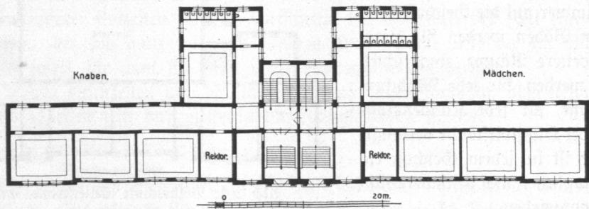
Abb. 205. Volksschule Barmbeckerstraße, Erdgeschoß.
