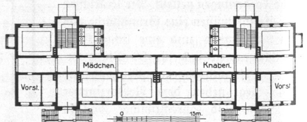
Abb. 204. Volksschule Ausschlägerweg, Erdgeschoß.
