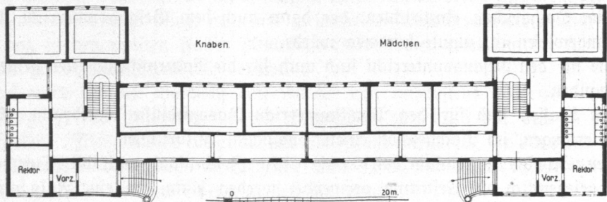
Abb. 206. Volksschule Rätbnerkamp, Erdgeschoß.
