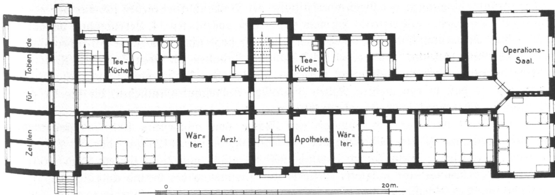
Abb. 198. 2. Gefängnis Fuhlsbüttel am Hasenberge, Lazarettgebäude, Grundriß, Erdgesch.ß.
