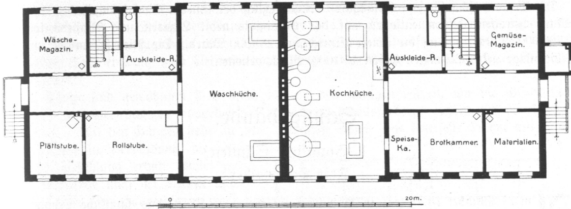
Abb. 197. 2. Gefängnis Fuhlsbüttel am Hasenberge, Küchengebäude, Grundriß, Erdgesch.ß.
