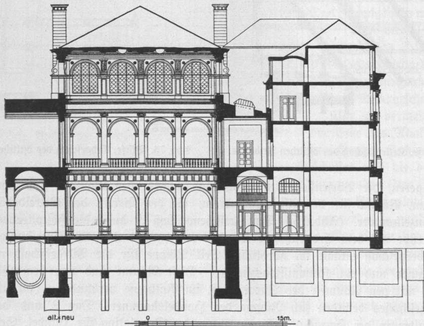
Abb. 77. Börse, Querschnitt durch den östlichen Anbau.
