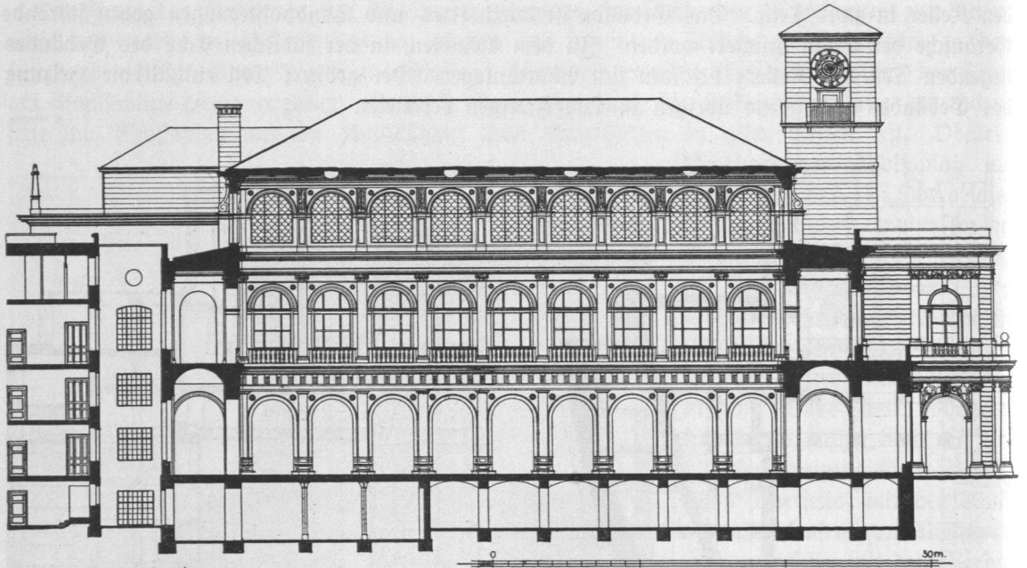
Abb. 76. Börse, Längsschnitt durch den östlichen Anbau.
