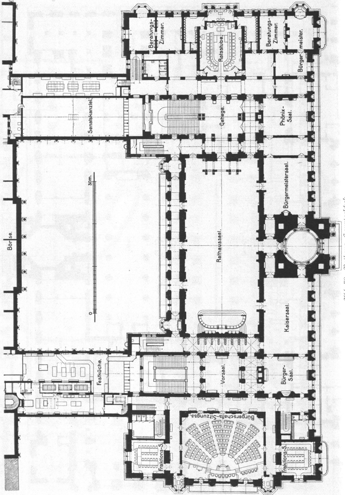
Abb. 70. Rathaus, Hauptgeschöß.
