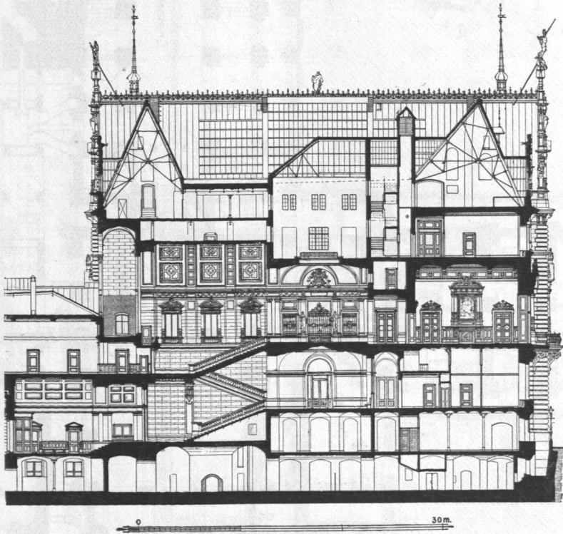
Abb. 67. Rathaus, Querschnitt durch die Senatstreppe.
