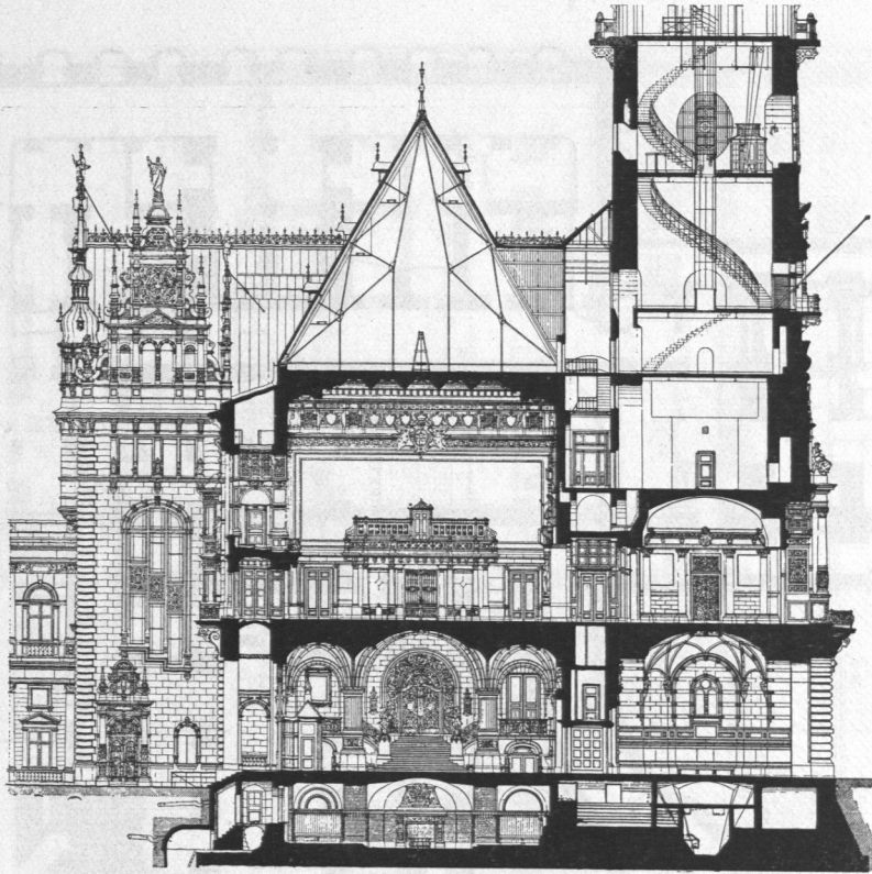
Abb. 66. Rathaus, Querschnitt durch den Turm.
