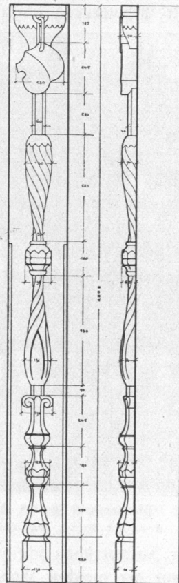
Abb. 35. Fachwerkständer im Museum für Hamburger Geschichte.
