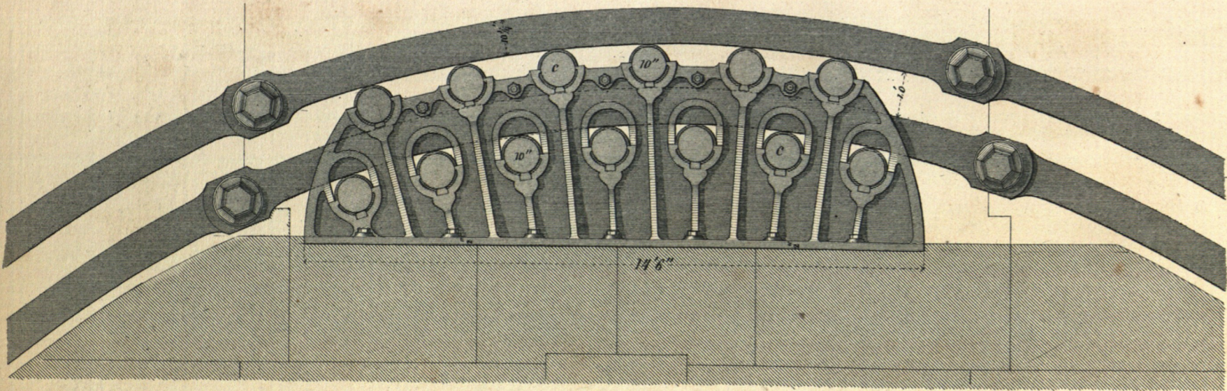
Fig. 12. Oberansicht der Lagerstühle.
