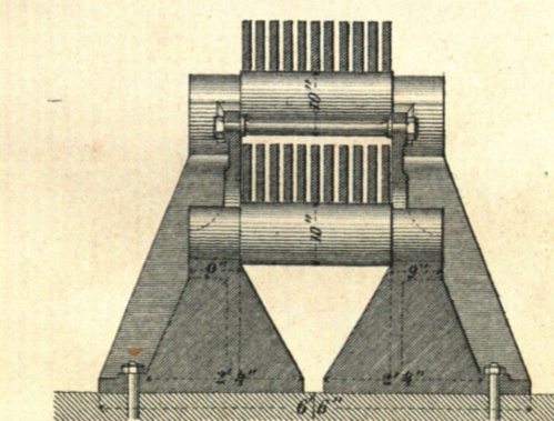
Fig. 13. Seitenansicht der Lagerstühle.
