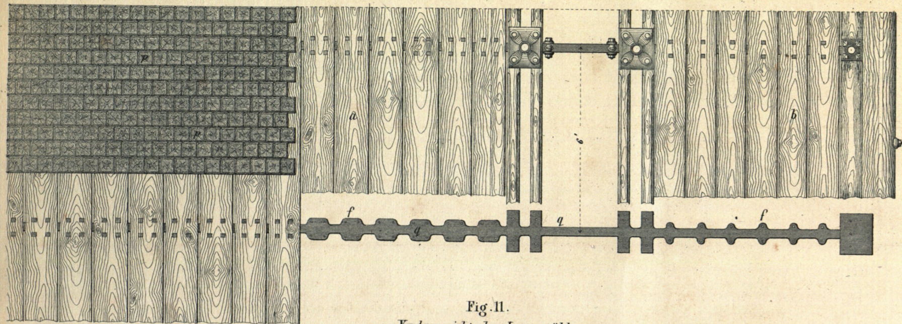
Fig. 6. Oberansicht der Brückenbahn u. des Querträgers.
