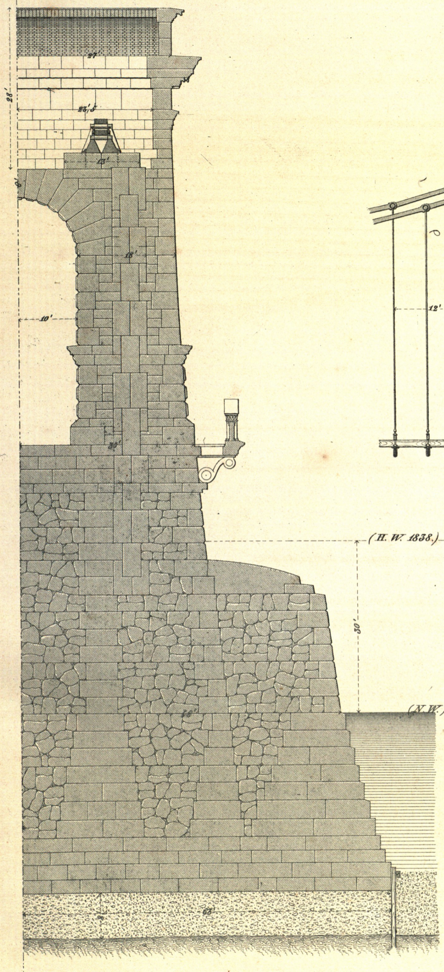
Fig. 3. Längenschnitt des Tragpfeilers.
