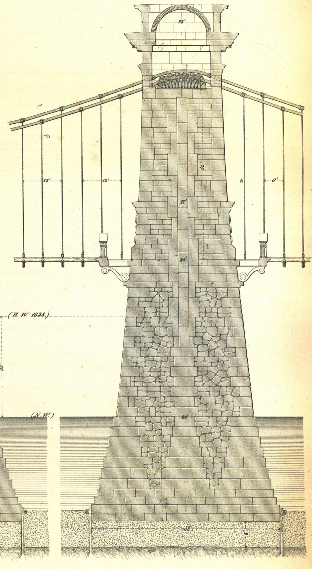
Fig. 4. Querschnitt des Tragpfeilers.
