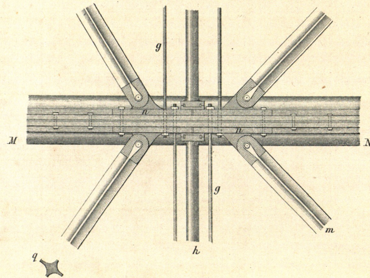
Zu Fig. 31 u. 32. 0 5 1 2 Meter.
