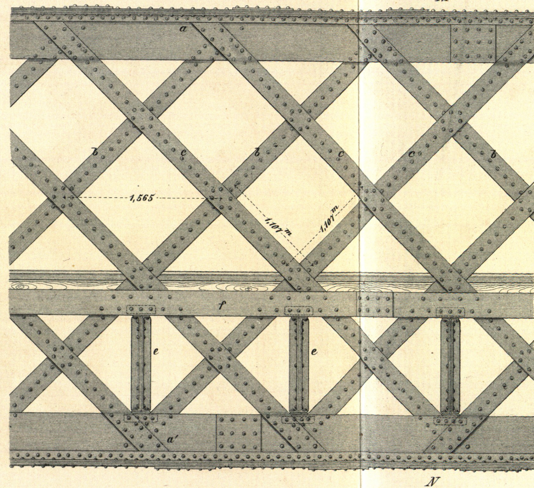
Ansicht der Mitte eines Hauptträgers.
