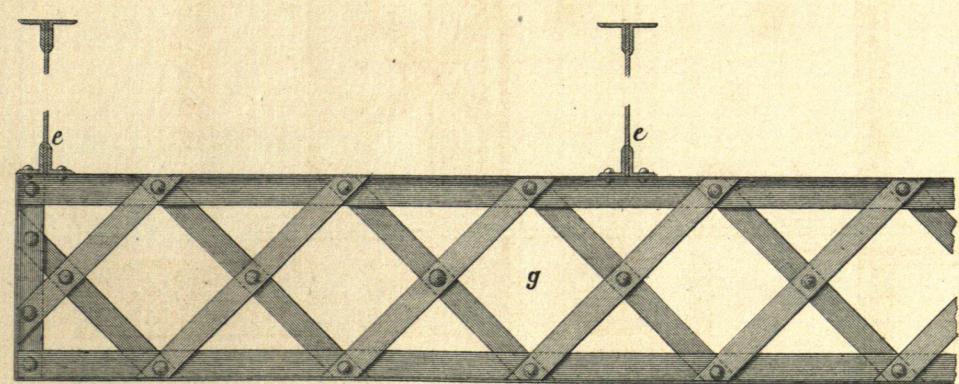
Durchzug unter den Querträgern der Hauptöffnung.
