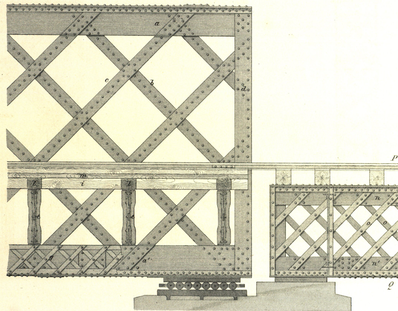
Längenschnitt und Anlager der Haupt- u. Seiten-Träger.
