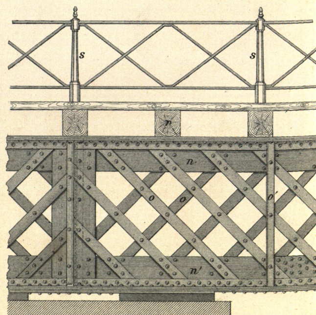
Ansicht eines Seitenträgers.
