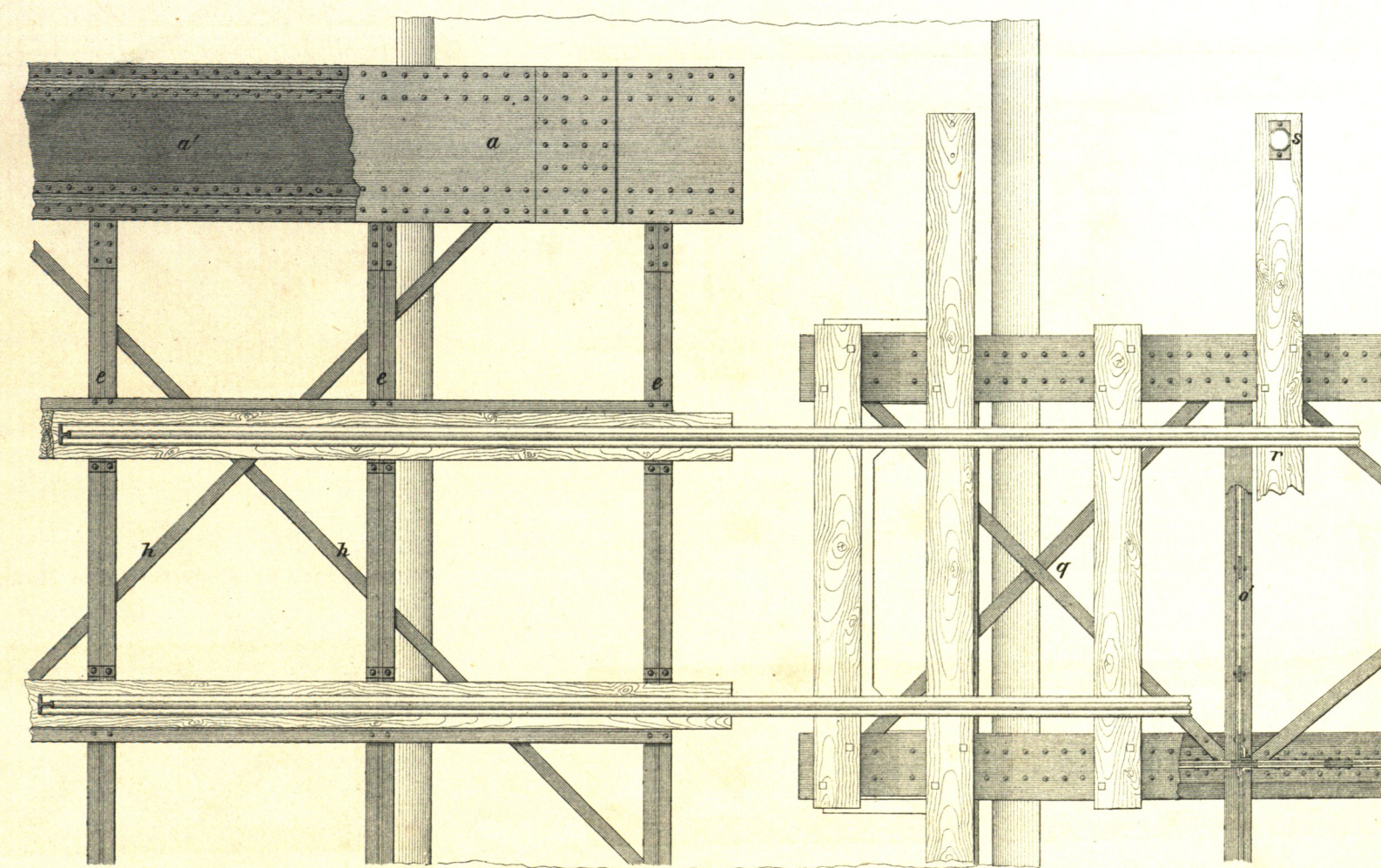
Grundriss zu Fig. 21.
