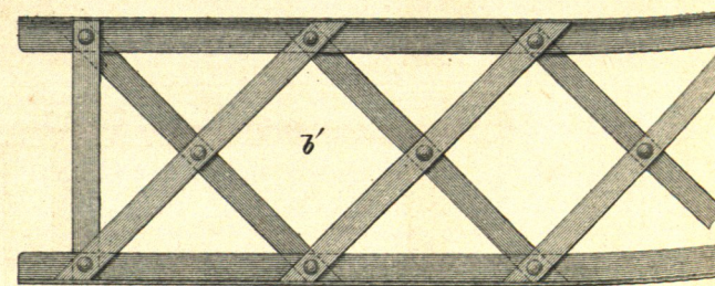
Diagonale Absteifung der Hauptträger.
