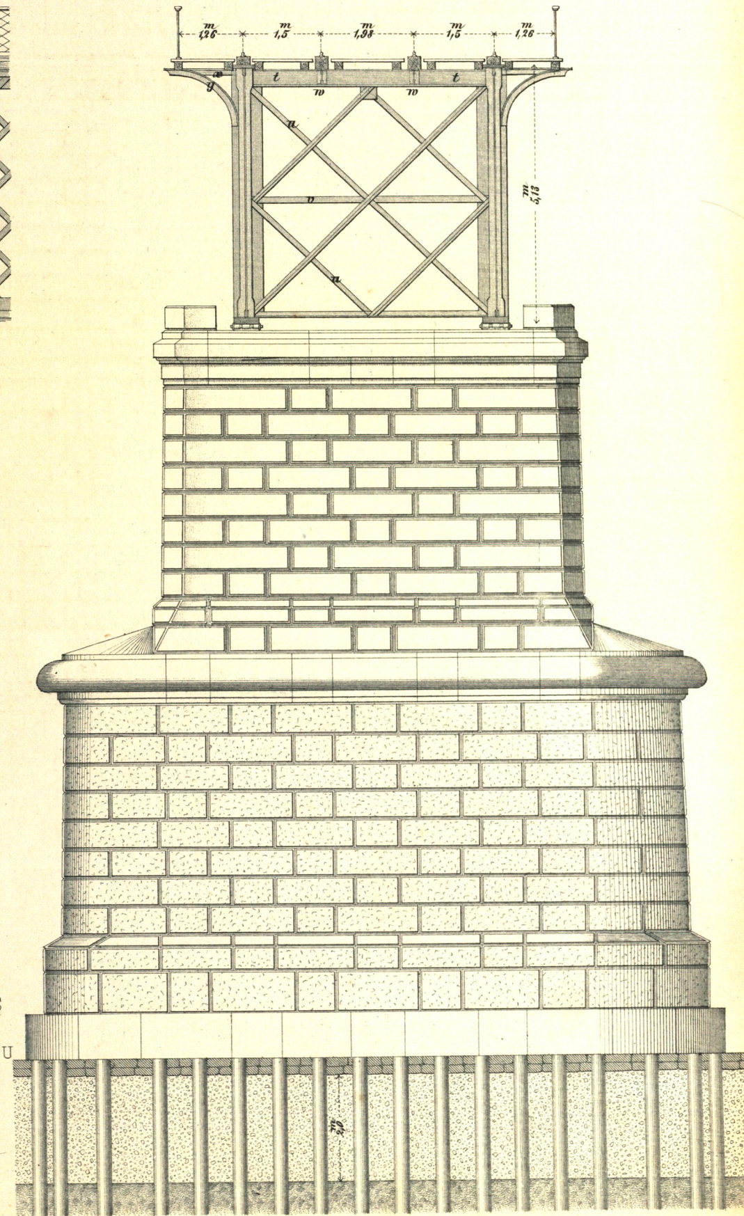
Seitenansicht eines Pfeilers.
