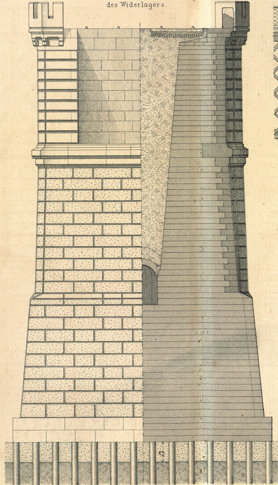
Seitenansicht u. Schnitt nach G-H des Widerlagers.
