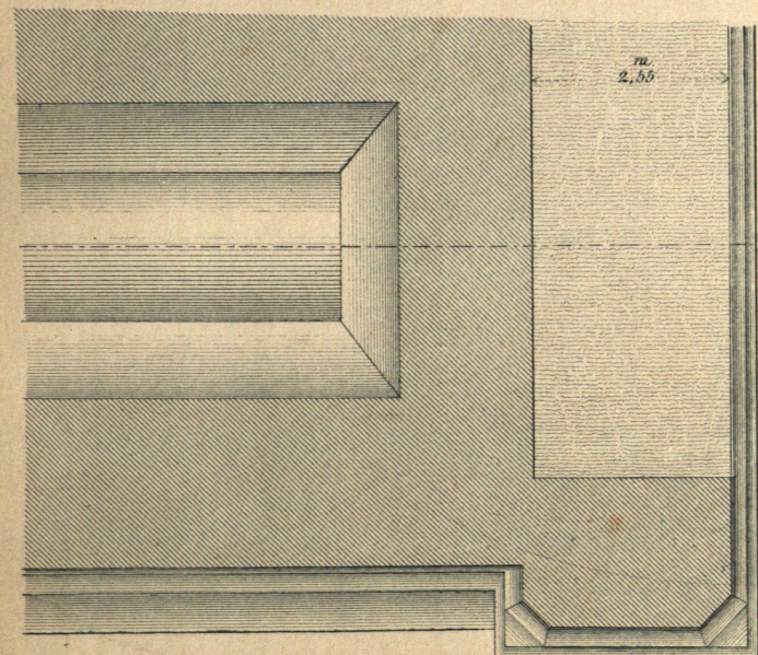
Grundriss des Widerlagers.
