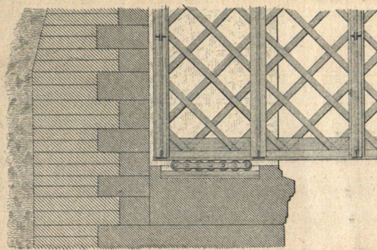
Schnitt durch das Widerlager u. Ansicht des Rollenlagers.
