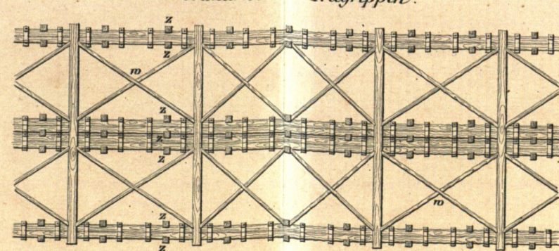
Fig. 4. Grundriss der Tragrippen.
