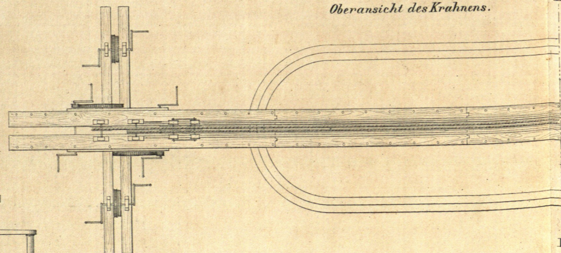
Fig. 3. Oberansicht des Krahnens.
