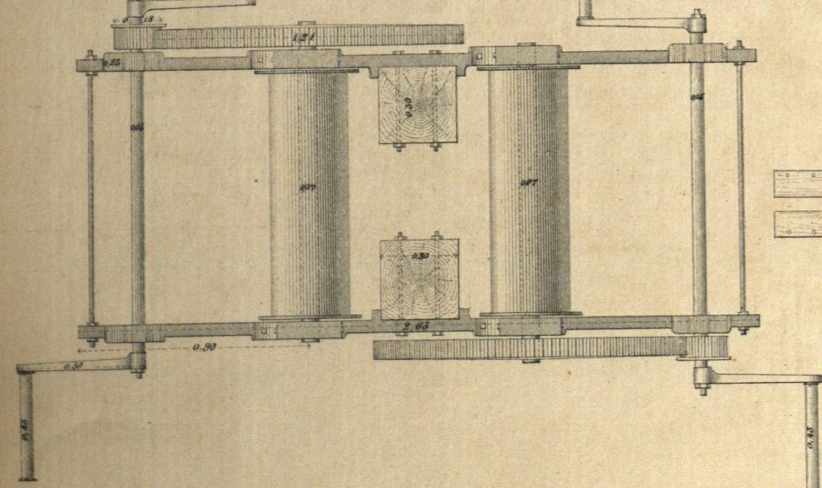
Oberansicht der Haspeln.
