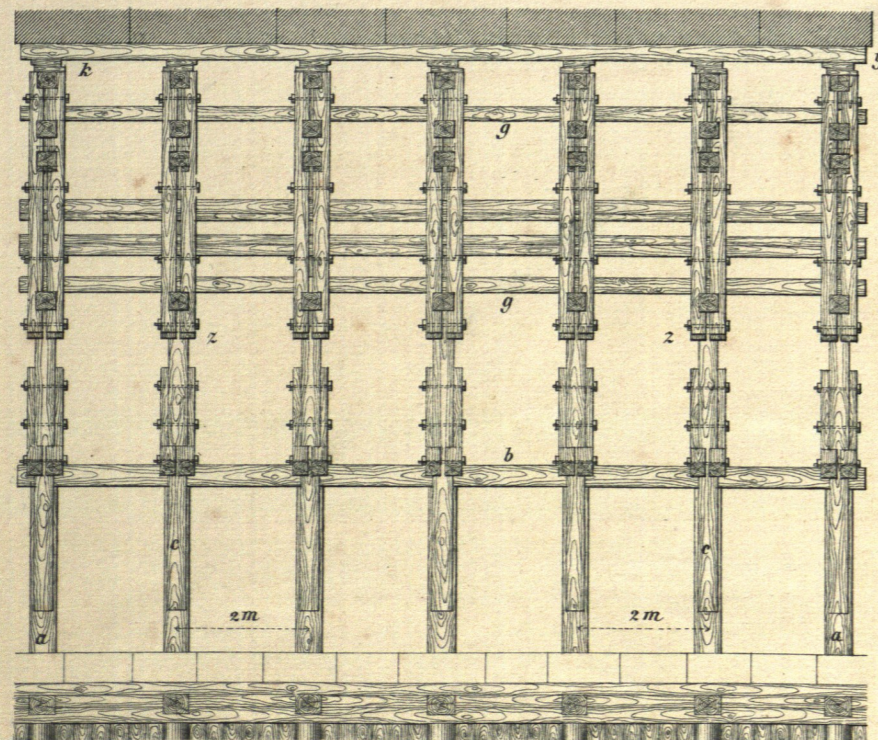
Fig. 3. Querschnitt nach C.D.
