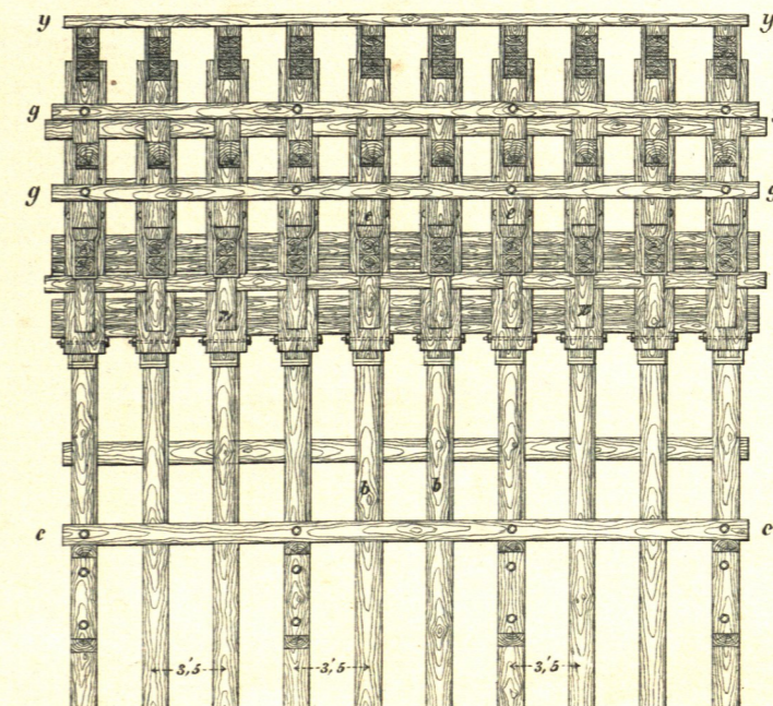
Fig. 6. Querschnitt nach E.F.
