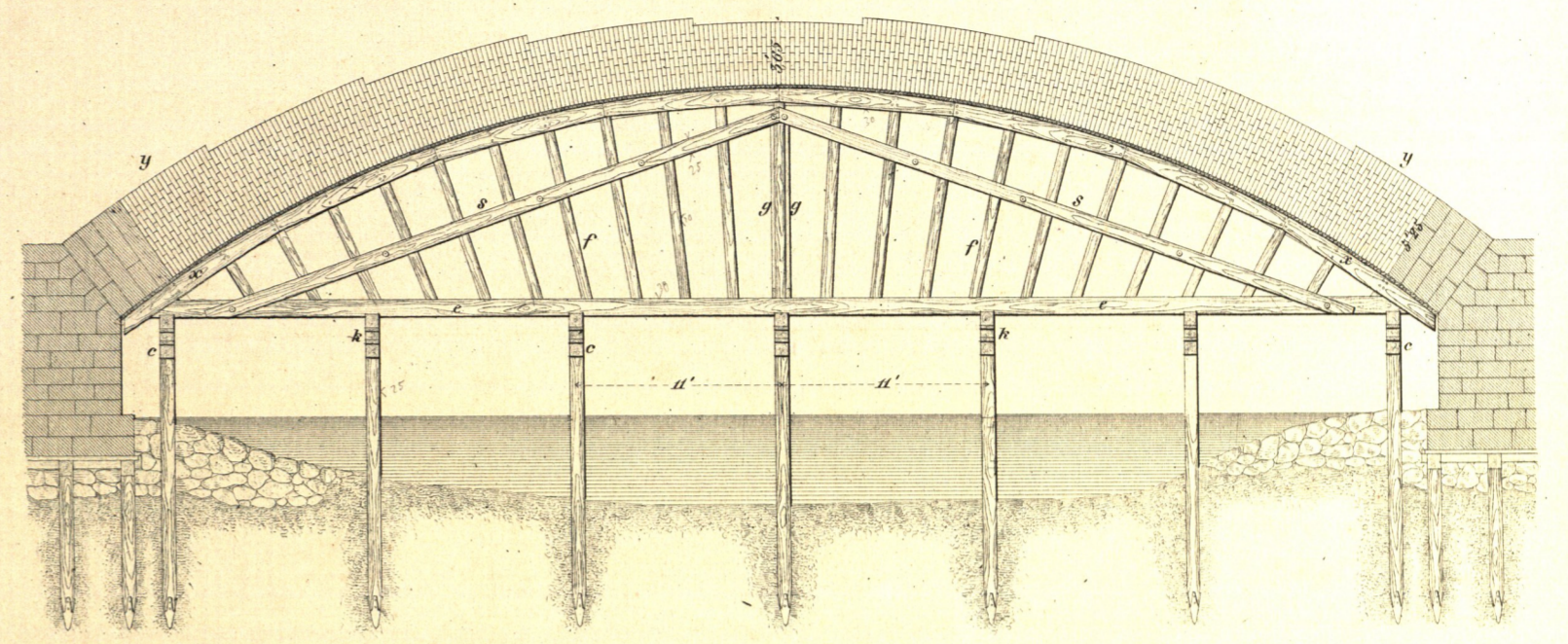
Fig. 4. Längenschnitt.
