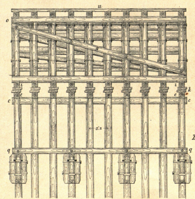
Fig. 3. Querschnitt nach E F.
