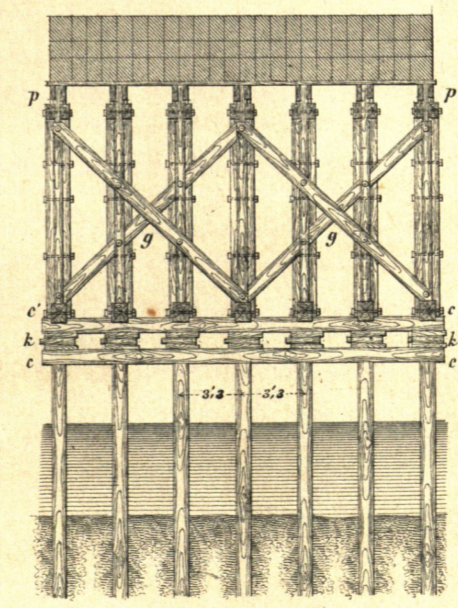
Fig. 6. Querschnitt nach GH.
