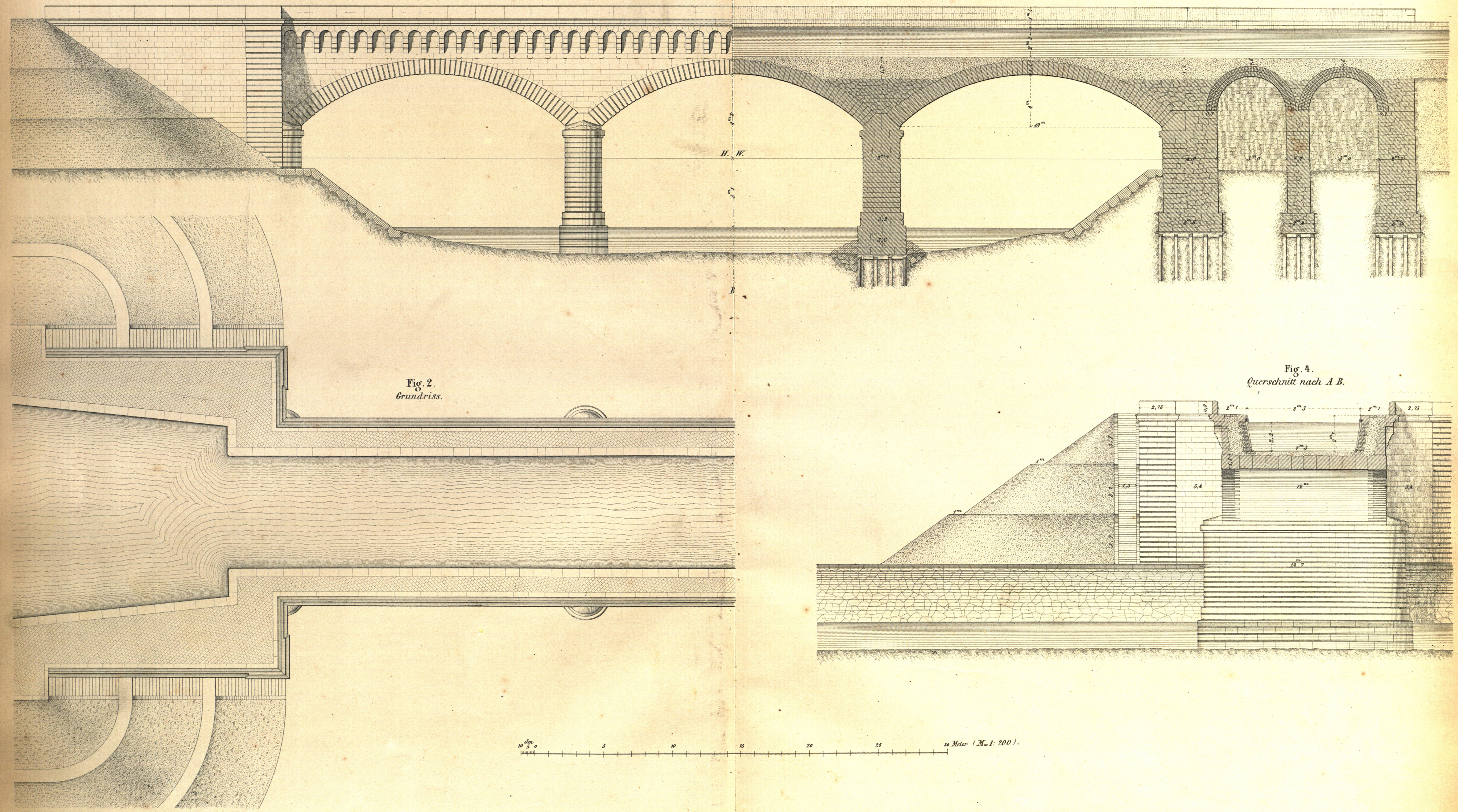
Fig. 1. Längenschnitt.
