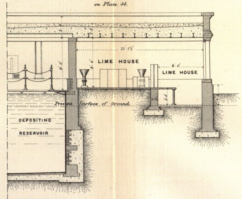
FIG. 3. Section N. O. on Plate 44.
