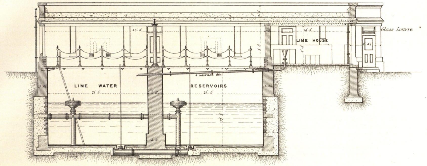
FIG. 2. Section L. M. on Plate 44.
