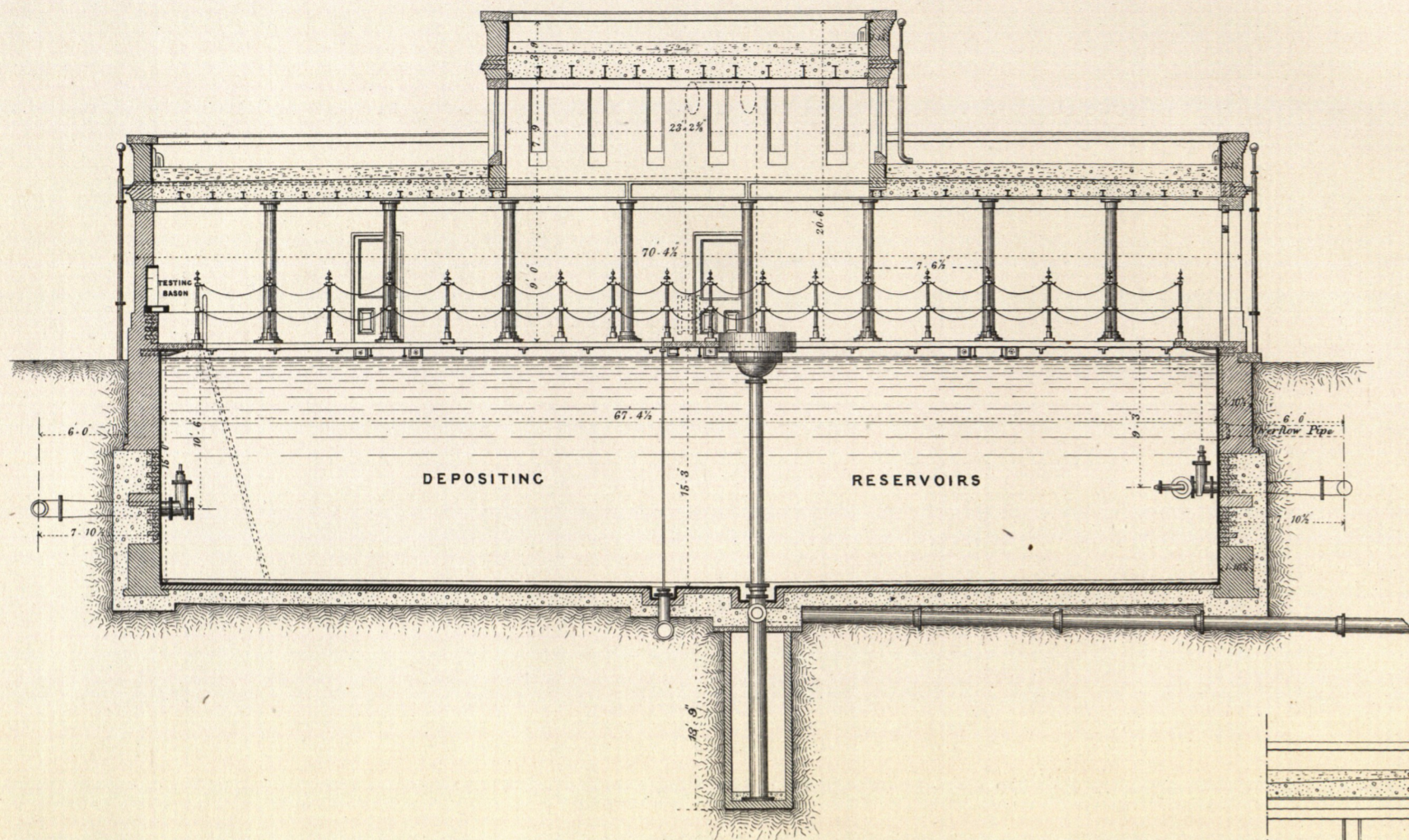
FIG. 1. Section I. K. on Plate 44.
