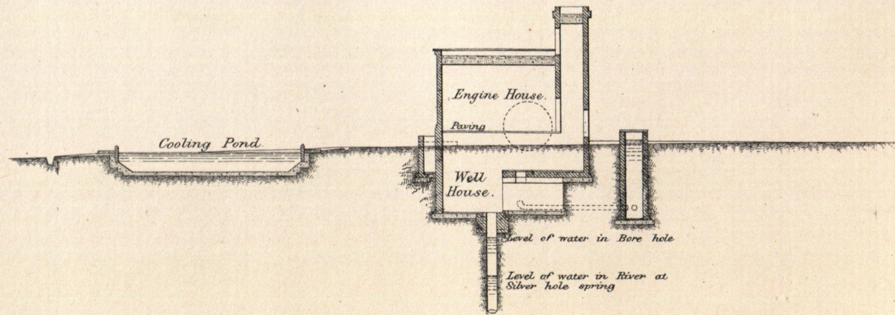
FIG. 5. Section C. H.
