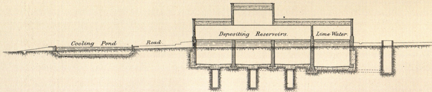
FIG. 4. Section E. F.
