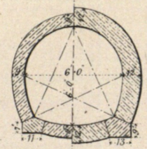
FIG. 15. Section A.B.
