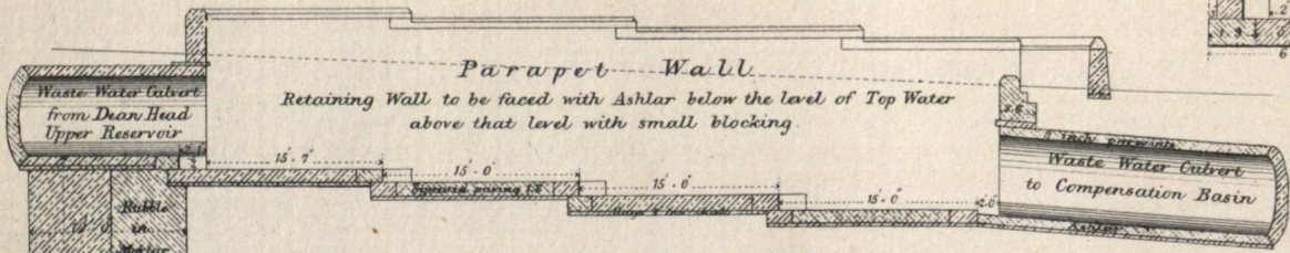
FIG. 4. Section P.Q.
