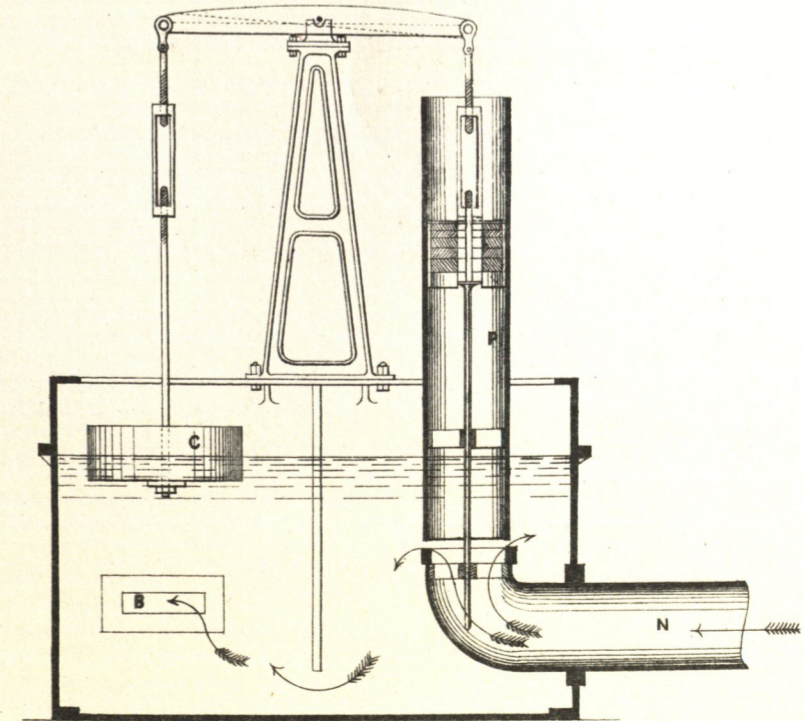
FIG. 15 Longitudinal Section
