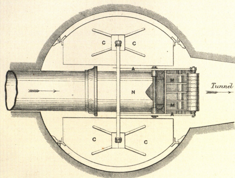
FIG. 13. Plan.
