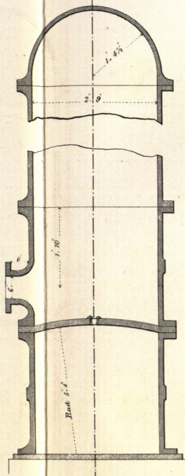
FIG. 6. Section A. A.
