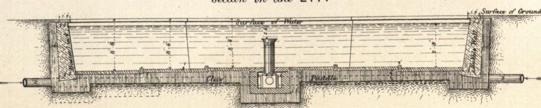
FIG. 4. Section on line E. F.
