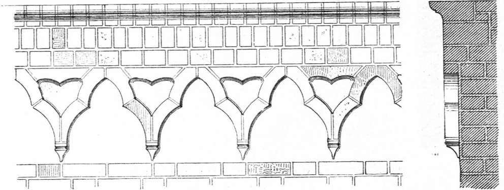
Hauptgesims an der Marienkirche zu Salzwedel 48) .
