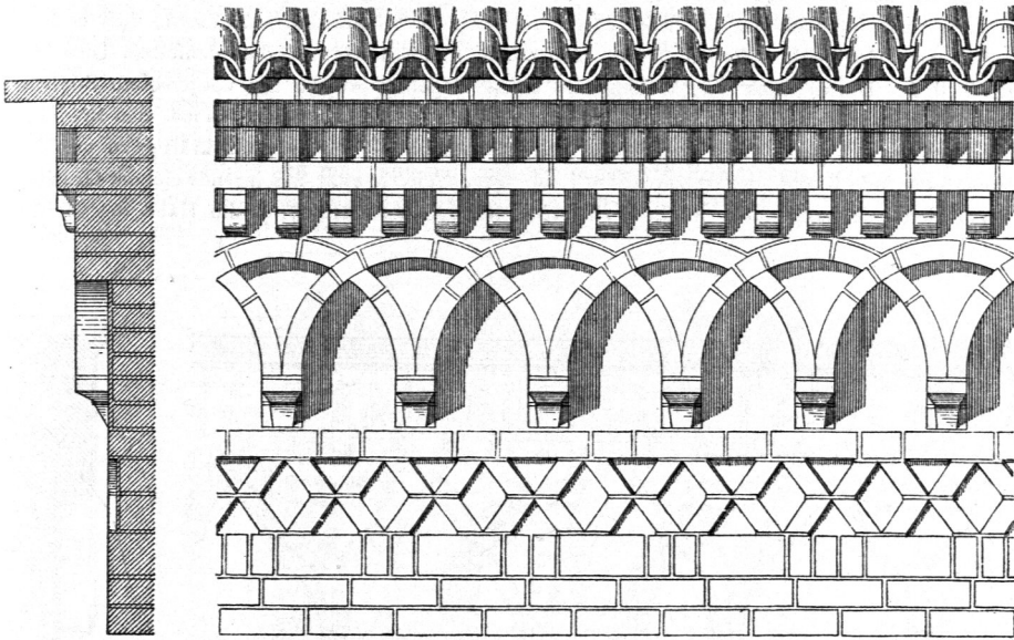
Hauptgefims an der Kirche Sant' Ambrogio zu Mailand 32 ).
