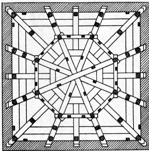
Grundriffe in der Höhe der wagrechten Balken.
