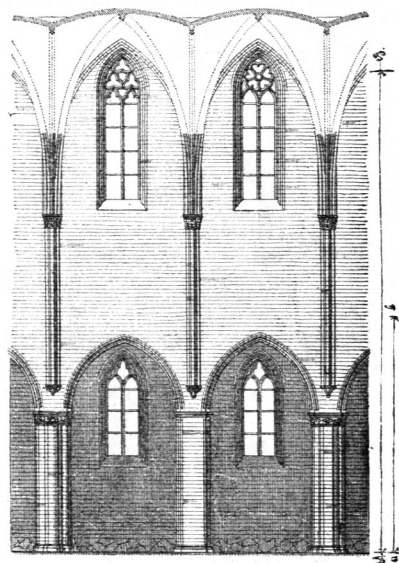
Längenschnitt.
