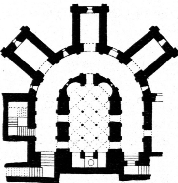
Kirche St.-Philibert zu Tournus. Grundriß der Krypta. — \frac{1}{500} w. Gr.
