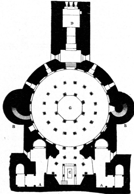
Kirche St.-Benigne zu Dijon. Grundriß der Krypta. — \frac{1}{500} w. Gr.
