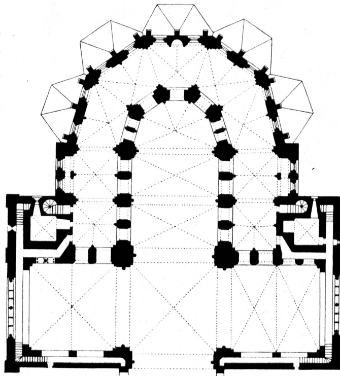
Oberer Chorgrundriß (Bischofsgang).
