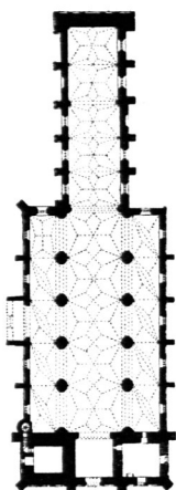
Dom zu Königsberg. Grundriß. 1/1000 w. Gr.
