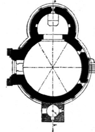
Grundriss. — \frac{1}{500} w. Gr. Karnen zu Mödling.
