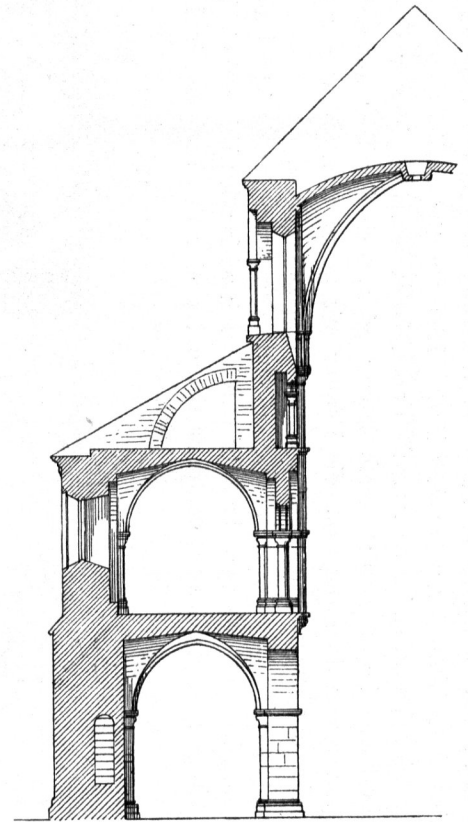
Querschnitt.
