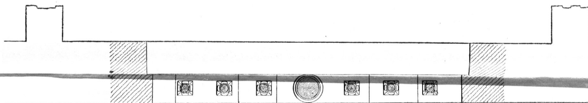
Südliche Mauer. — Grundrifs des Obergeschosses.
