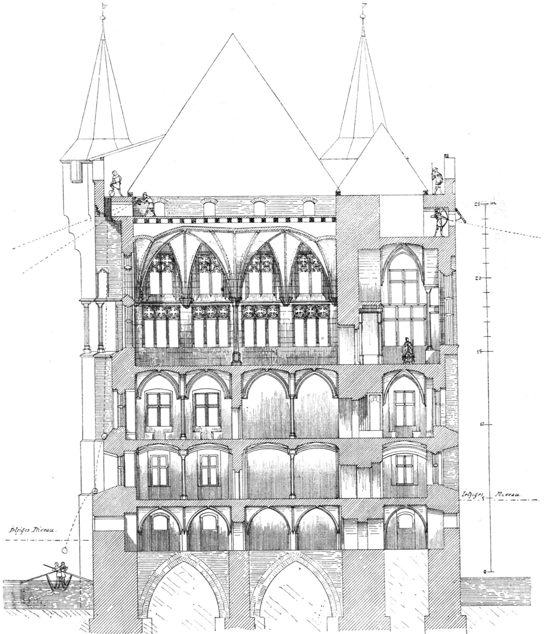
Schnitt.
