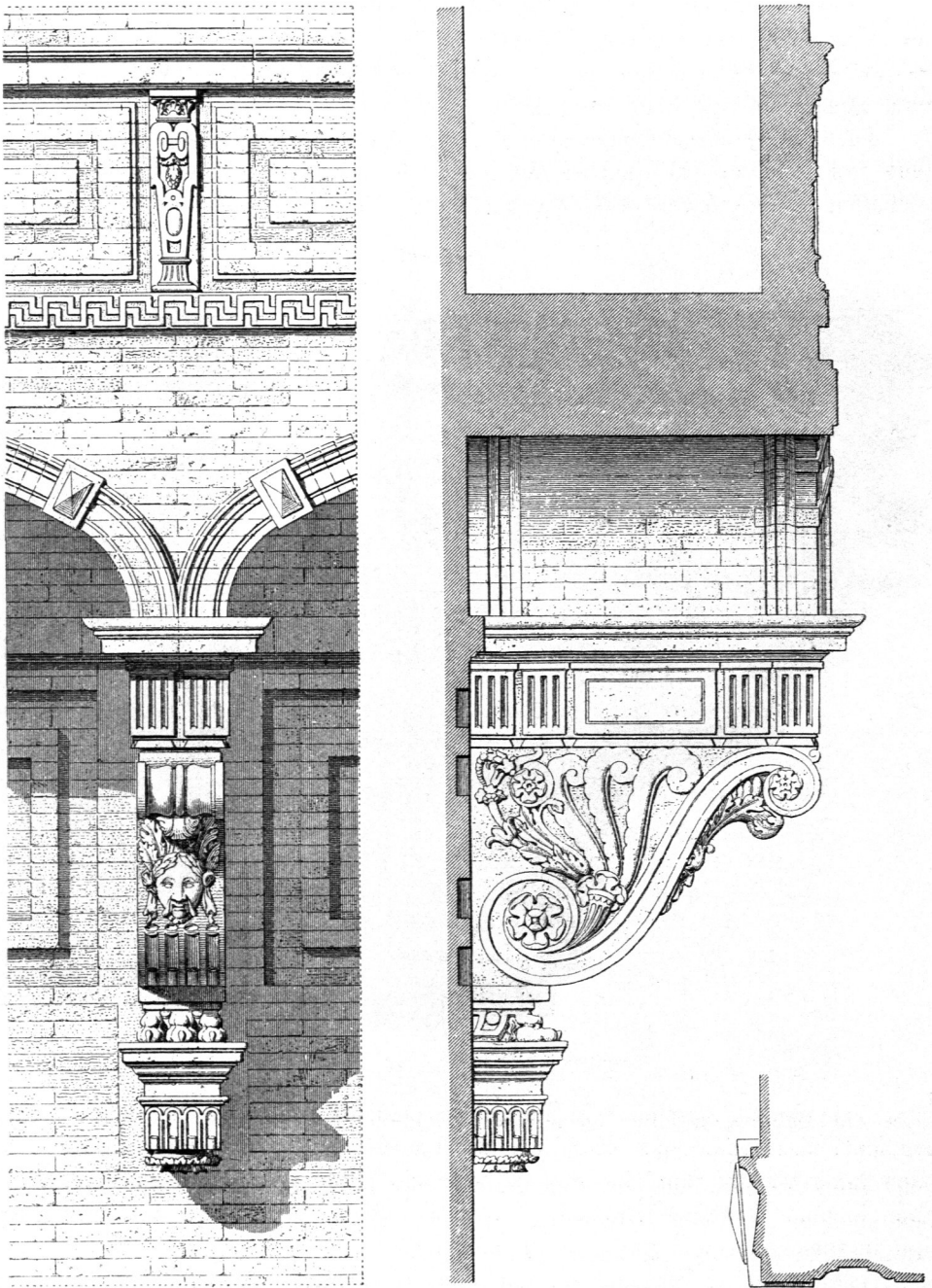
Tragstein unter einer Galerie im Hôtel d'Asszat zu Toulouse 118 ).
