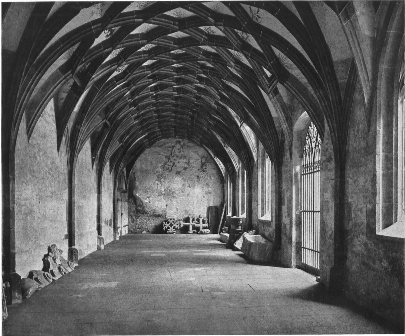
Kloster Maulbronn. — Das „Parlatorium“, der Sprechsaal, 1493 (Bf. = 5,7 × 25,2 m H. etwa 5,5 m)
