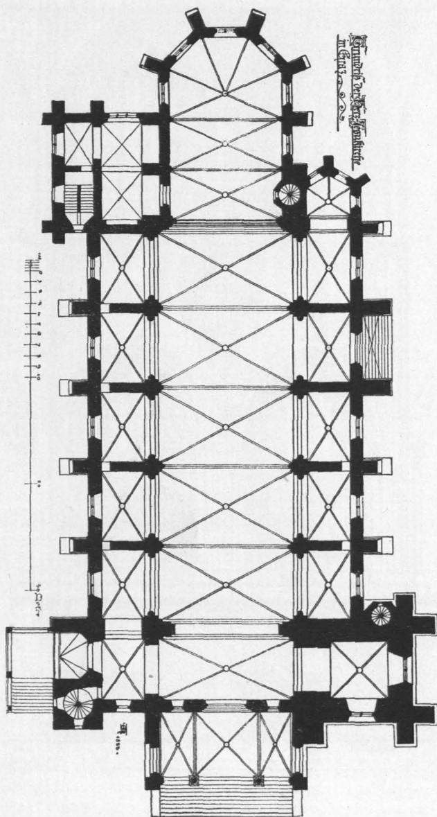
Tafel I. Grundriss der Herz-Jesu-Kirche. (Sieh S. 20.)
