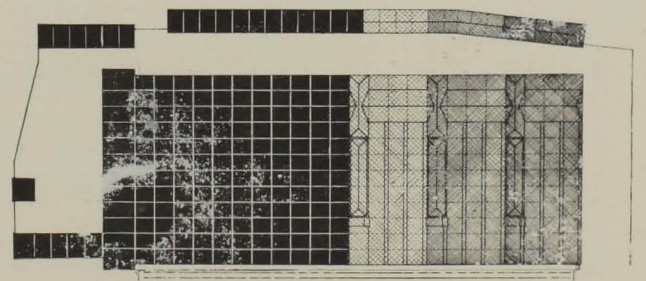
Abb. 61. 3. BAUABSCHNITT mit 3., 4. und 5. Erweiterung. Vollausbau wie Abb. 58
