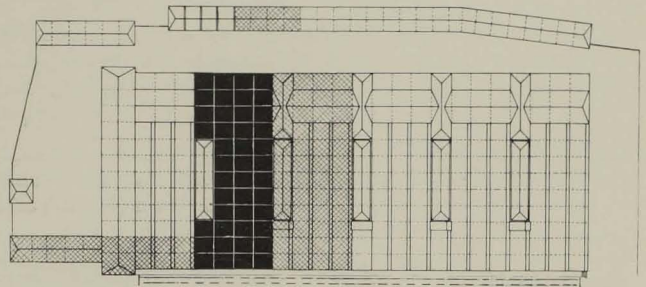
Abb. 58. LAGEPLAN ZU ABB 49. Neugestaltete Anlage, klarer, organischer Aufbau des Herstellungsprozesses im Baukörper. Typische Merkmale: Erst planmäßige Gesamtgröße, dann 1. Bauteil, umgekehrter Weg wie bei Abb. 50-57.
