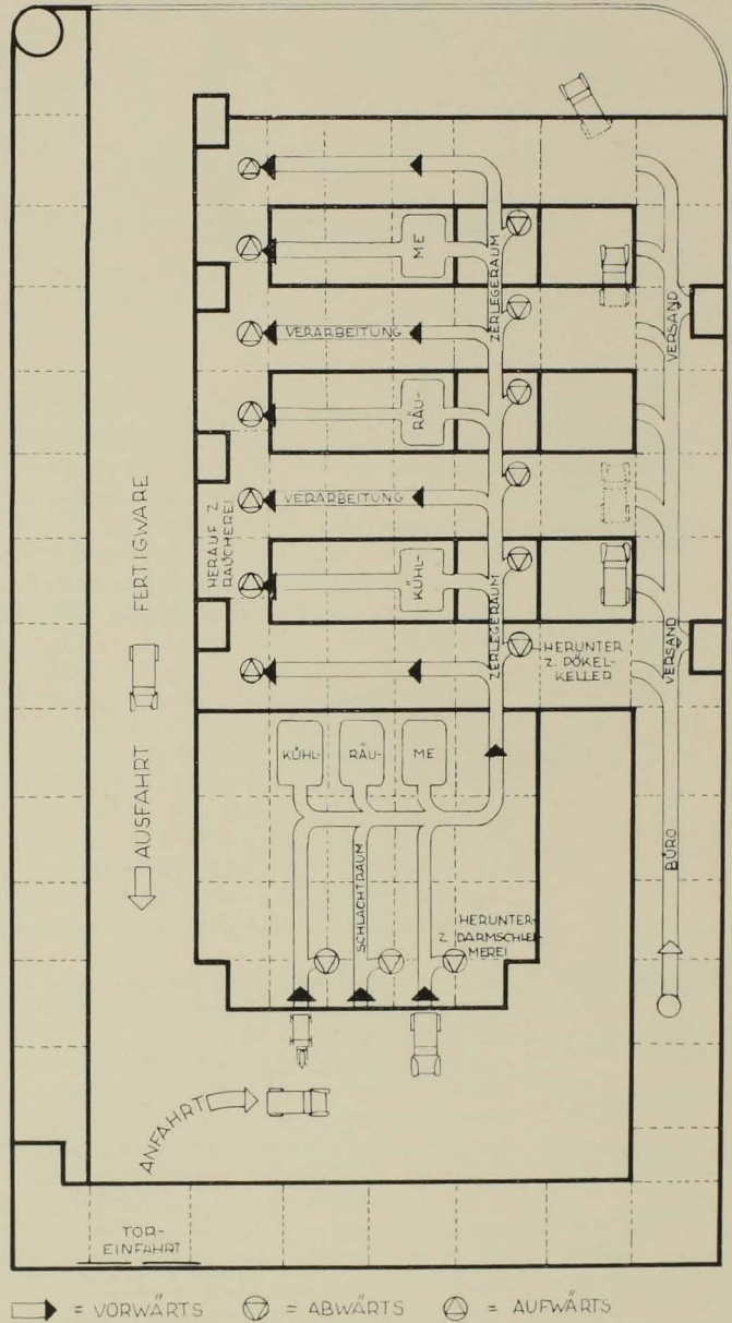
Abb. 45. ENDGÜLTIGER ORGANISATIONSPLAN der Gesamtanlage. Verkleinerte Anlage gegenüber Organisationsplan Abb. 5. Die Verkleinerung der Anlage wurde mit Rücksicht auf die derzeitigen Dezentralisierung vorgenommen. Auf Grund der Erfahrung im 1. Bauteil hat sich ergeben, daß die Verkürzung der Verarbeitungswege günstiger ist.
