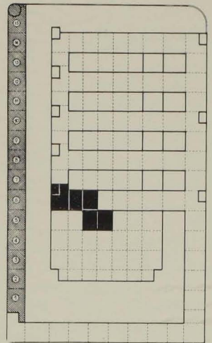
Abb. 44. ZELLENAUF- BAU des Nebenraumes
