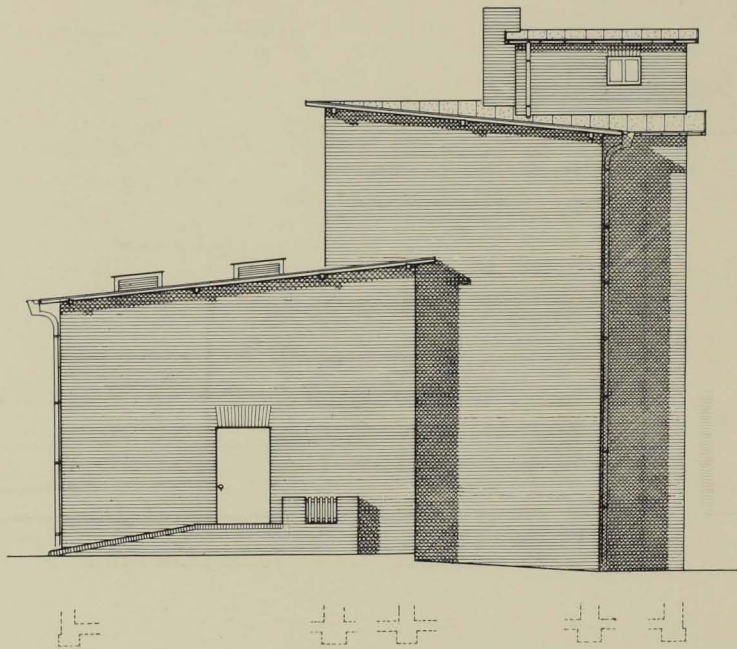
Abb. 32. OSTANSICHT, AUSFÜHRUNGSPLAN des 1. Bauteiles der W. F. F.
