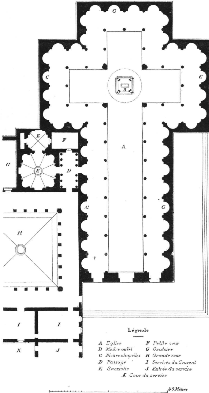
PLAN DE L'ÉGLISE ET DE LA SACRISTIE DE SAN-SPIRITO
