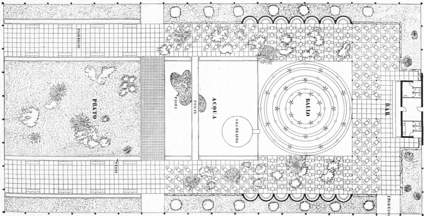
Das Gartenrestaurant im Modopalast in Turin. Blick auf den Orchesterplatz und die beleuchtete Bar. Grundriß 1:500. Architekt Ettore Sotsas, Turin
