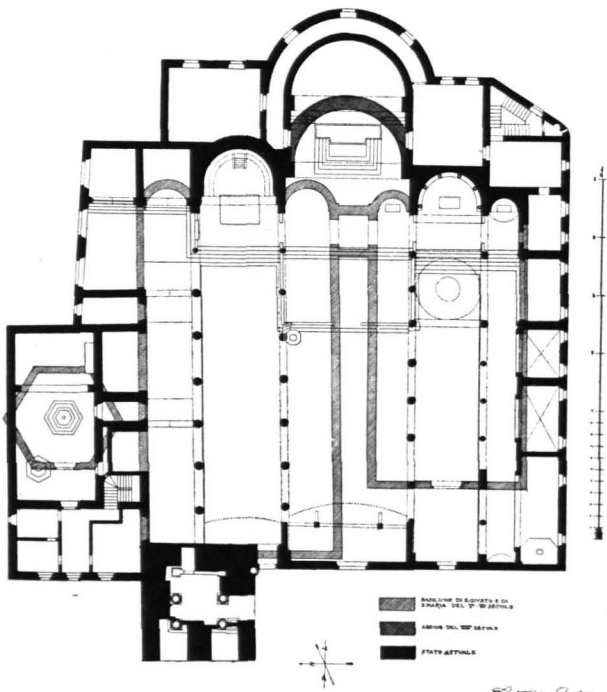
PIANTA CRONOLOGICA DELLA BASILICA DI S. GIUSTO.
