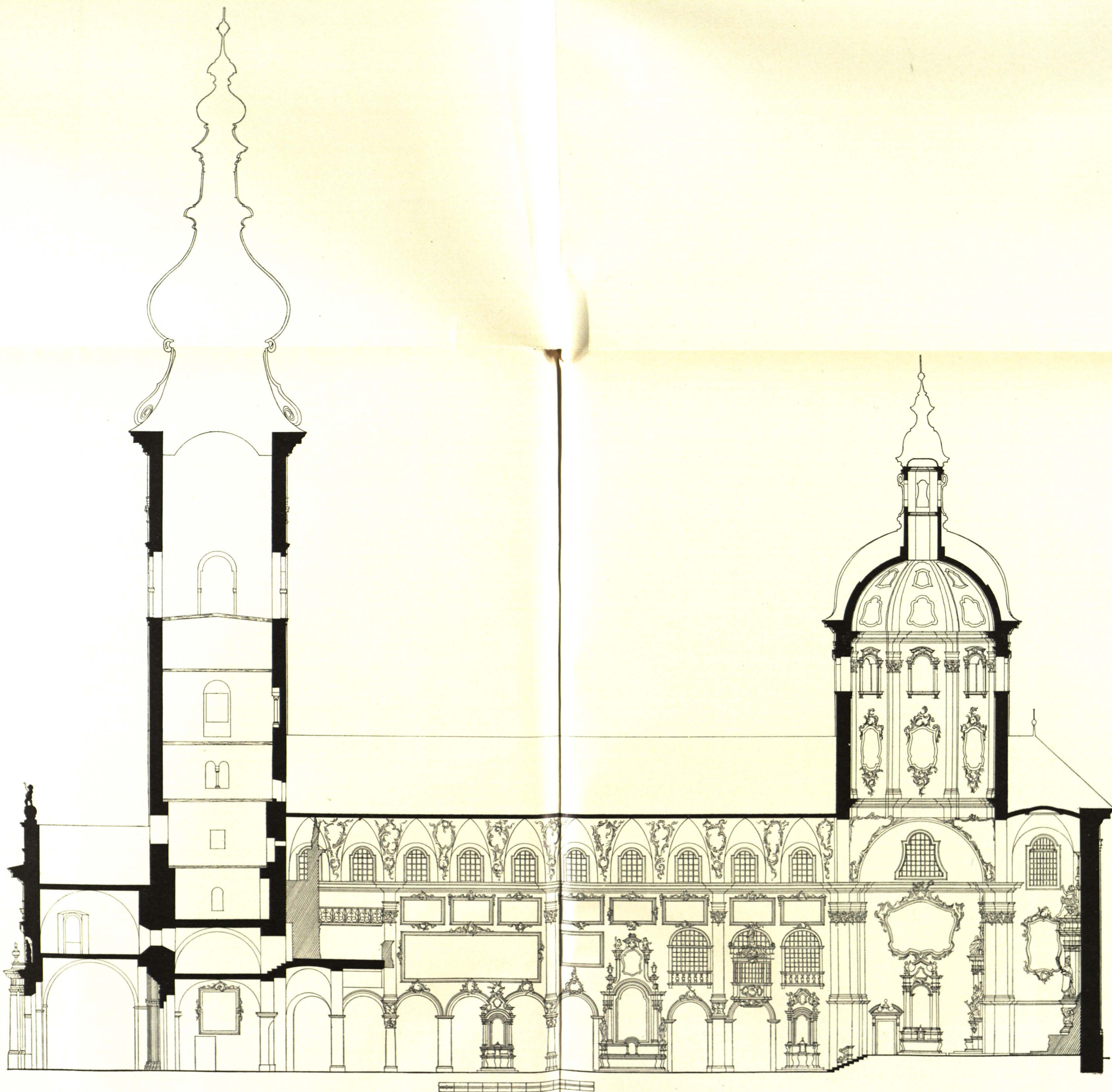
TAFEL II STIFTSKIRCHE, LANGENSCHNITT 1:200 (S. 2)
