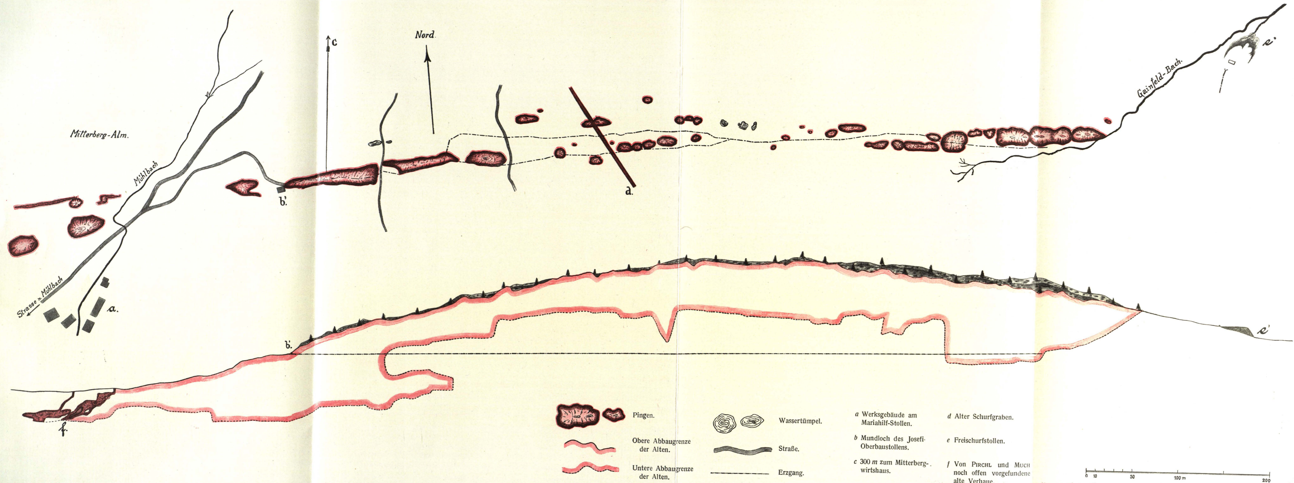
Fig. 1 Grund- und Aufriß der Pingen und des Abbaufeldes auf der Mitterbergalpe. (Nach einer bei der Gewerkschaft Mitterberg liegenden alten Grubenkarte.)
